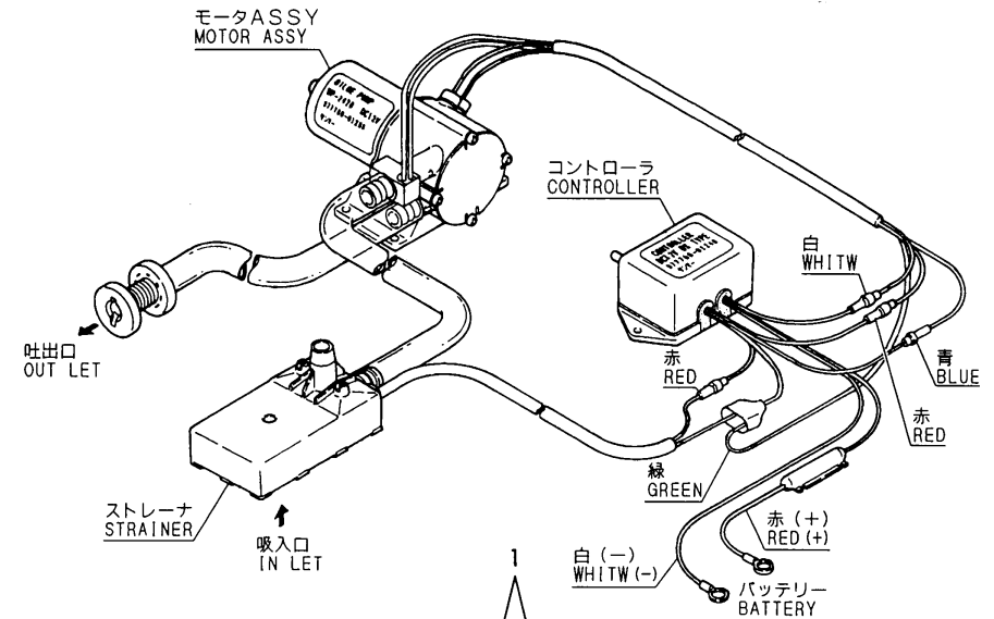
Fig.67. BILGE PUMP(DX,OPTIONAL)
